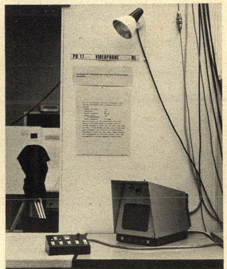
Bild 5. Fernsehtelefon Videophone. Vidicon-Kamera und Lautsprecher sind im Bildröhrengehäuse untergebracht, das Mikrofon steckt im Bedienungskästchen links. Diese Aufnahme zeigt den typischen Aufbau aller ausgestellten 110 Forschungsarbeiten
