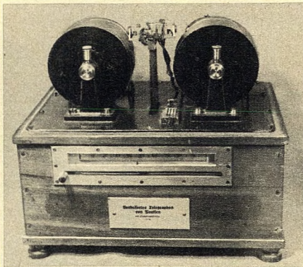
Bild 4. Verbessertes Poulsen-Telegraphon für Schnelltelegrafieempfang mit zwei Spulen für Stahldrahtstreifen (1904)
