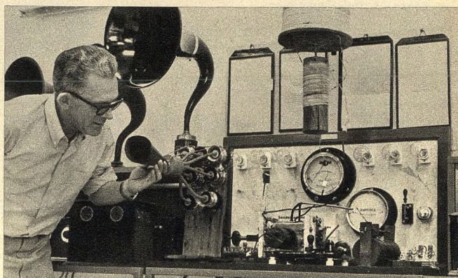
Bild 1. Der erste Telefonesender von Poulsen in Laboratoriumsausführung. In der Mitte die Flammenkammer mit Rohren für die Wasserstoffversorgung, davor eine Spule des magnetischen Gebläses, links das unmittelbar in die Antenne geschaltete Siebenfach-Kohlemikrofon
