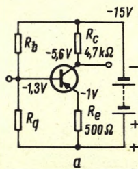
Bild 14. Verstärkerstufen mit Germanium-pnp-Transistor (a) und Silizium-npn-Transistor (b)
