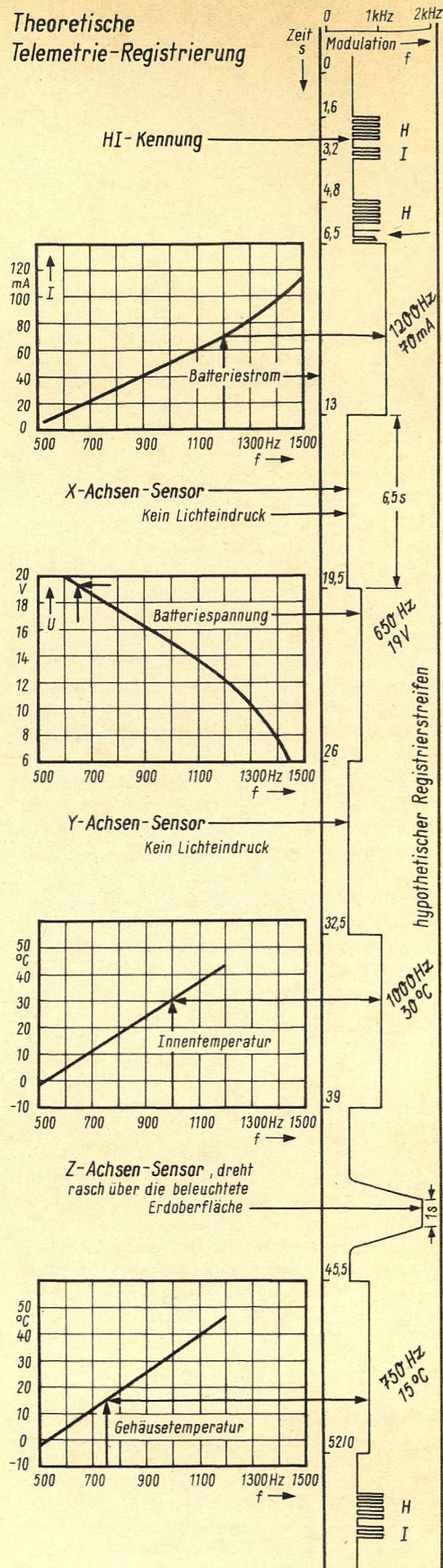
Rechts: Bild 2. Darstellung eines theoretischen Registrierstreifens zur Verdeutlichung des amateurnmäßigen Hörempfangs, mit Auswertung zur Eintragung in den von der Amsat herausgegebenen Telemetrie-Logbögen
