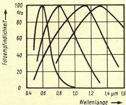
Kurven von Chalkogeniden-Gläsern unterschiedlicher Zusammensetzung. Durch Wahl der Glas-sorte läßt sich die maximale Fotoempfindlichkeit für bestimmte Längenwellenbereiche erzielen
