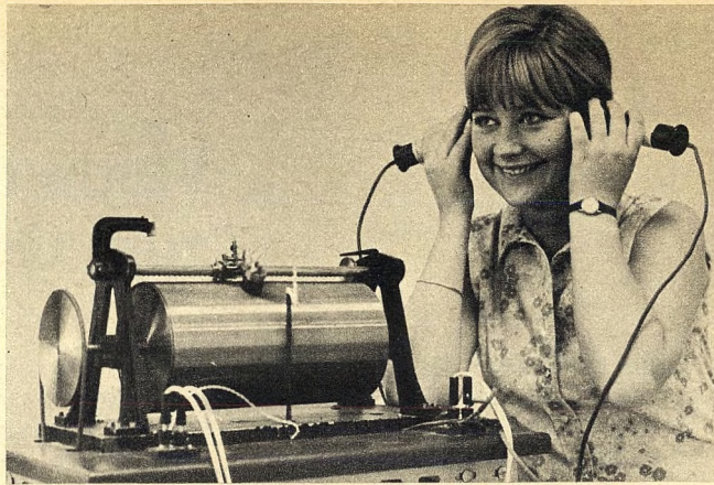
Bild 3. Poulsens erstes Telegraphon (1898) mit einer Drahtgeschwindigkeit von 2 m/s (DRP 109 569)
