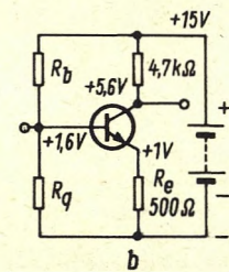
Bild 14. Verstärkerstufen mit Germanium-pnp-Transistor (a) und Silizium-npn-Transistor (b)
