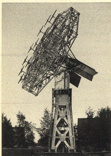
Bild 4. VHF-Spezialantennen für die unbemannt betriebenen Telemetriestationen Kevo, Reykjavik und Ft. Churchill
