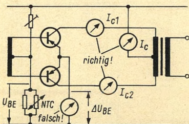
Messen von Ruhestromen in einer Gegentakt-B-Schaltung
