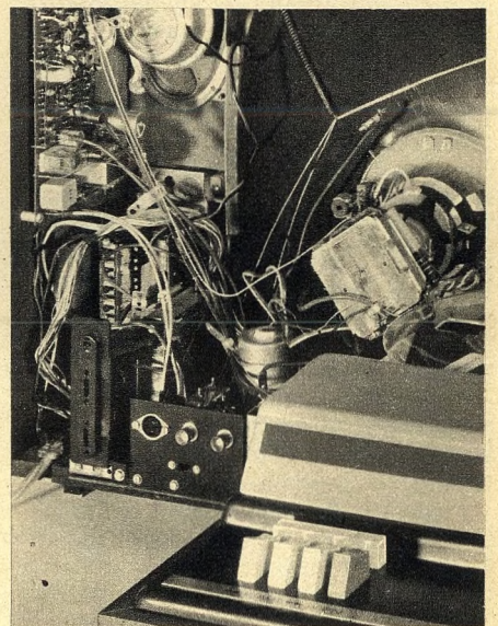
Links: Bild 8. Platine mit den Bauelementen des Videotransformators
