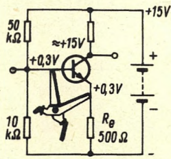
Bild 15. Prüfung der Steuerwirkung
