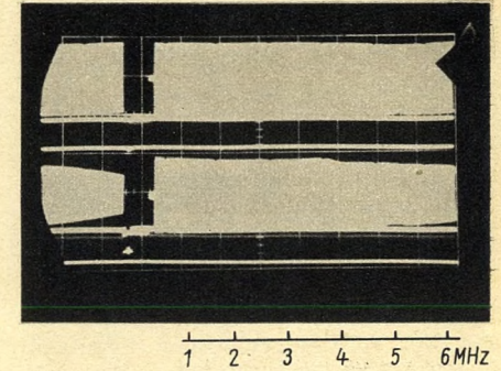
Bild 7. Frequenzgang des Eingangssignals, 1 V/cm und 2 ms/cm, jede Marke 1 MHz höher (oben). Frequenzgang des Ausgangssignals, zweimal über Videotransformator, 1 V/cm und 2 ms/cm (unten)
