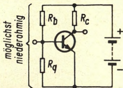
Bild 12. Basisspannung durch Spannungsteiler erzeugt
