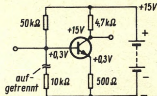
Bild 17. Spannungen an den Elektroden bei kurzgeschlossener Basis-Emitter-Strecke
