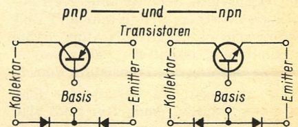
Bild 5. npn- und pnp-Transistoren
