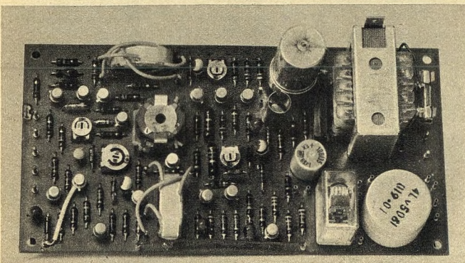
Links: Bild 8. Platine mit den Bauelementen des Videotransformators
