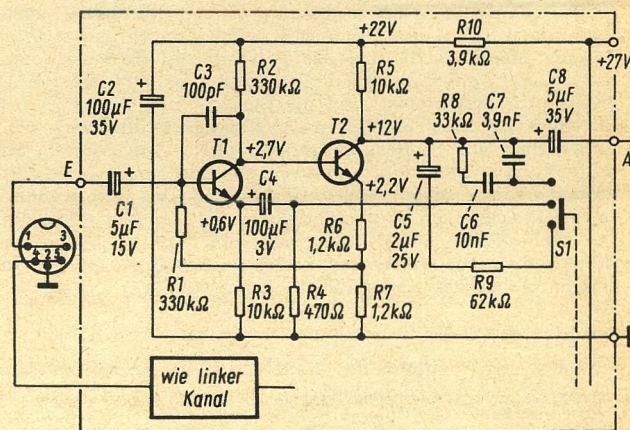
Schaltung der umschaltbaren Stereo-Vorverstärkerbaugruppe
